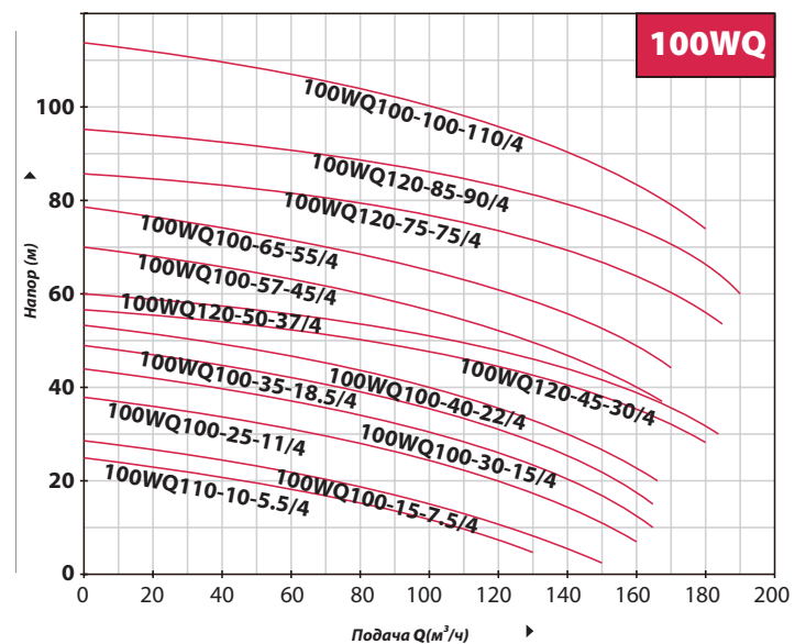
Кривая производительности
