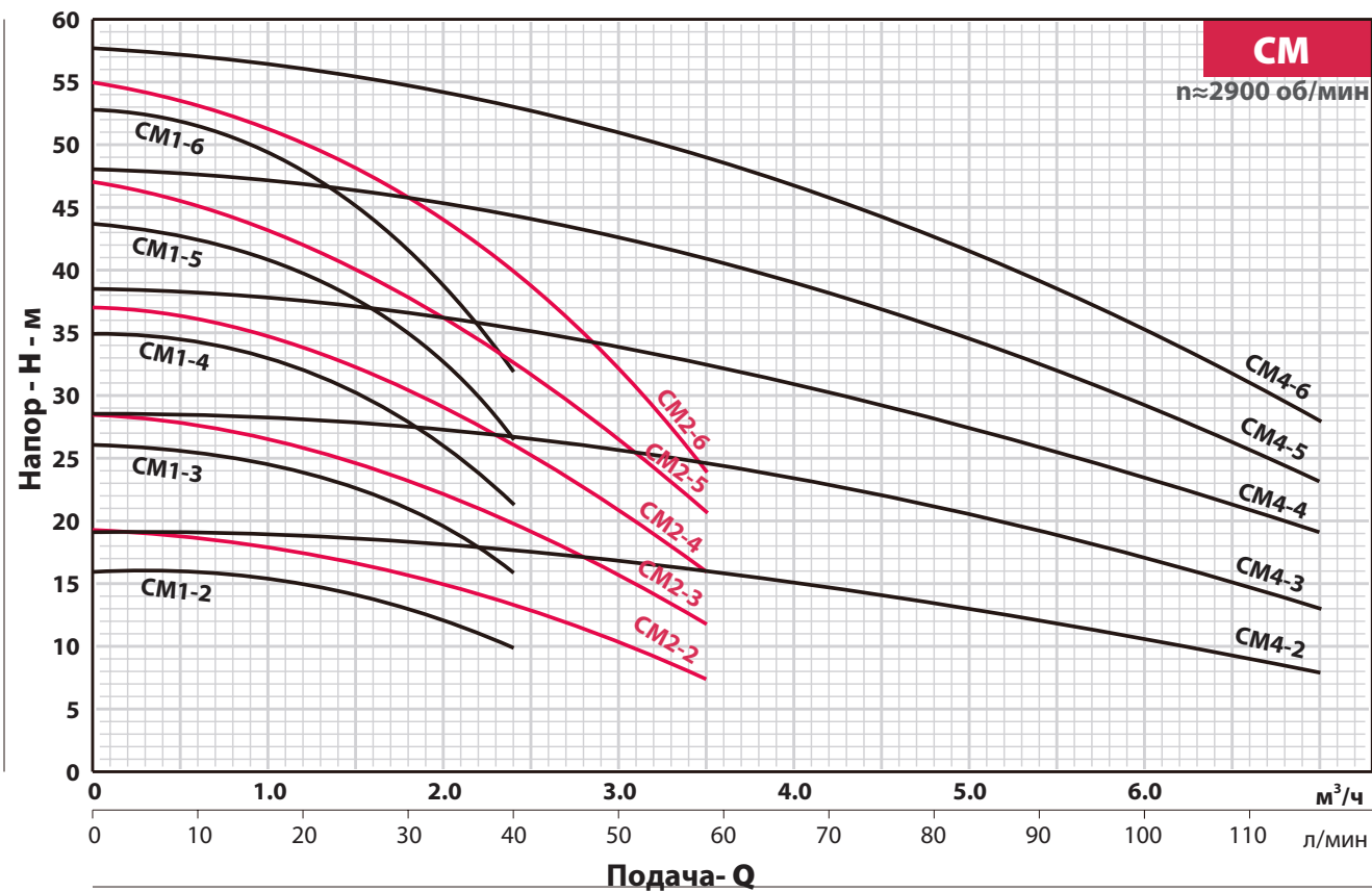
Кривая производительности
