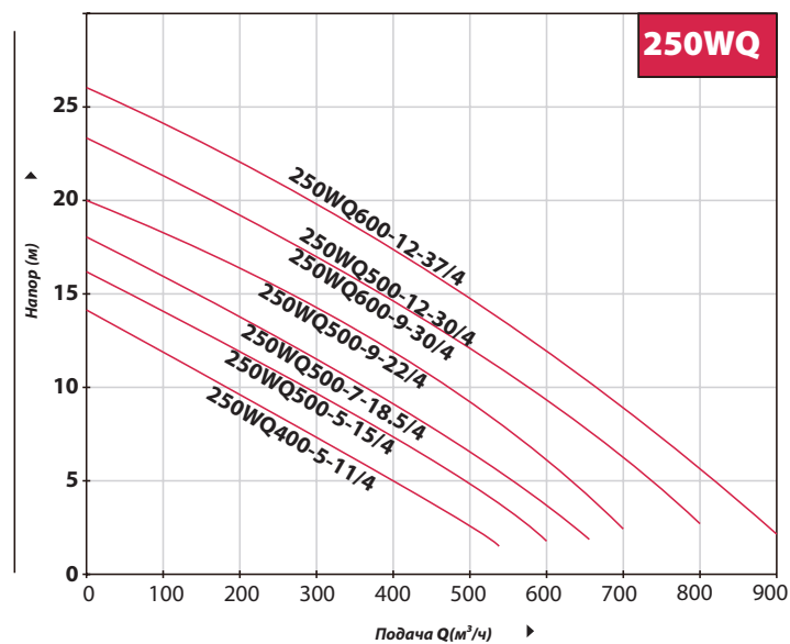
Кривая производительности
